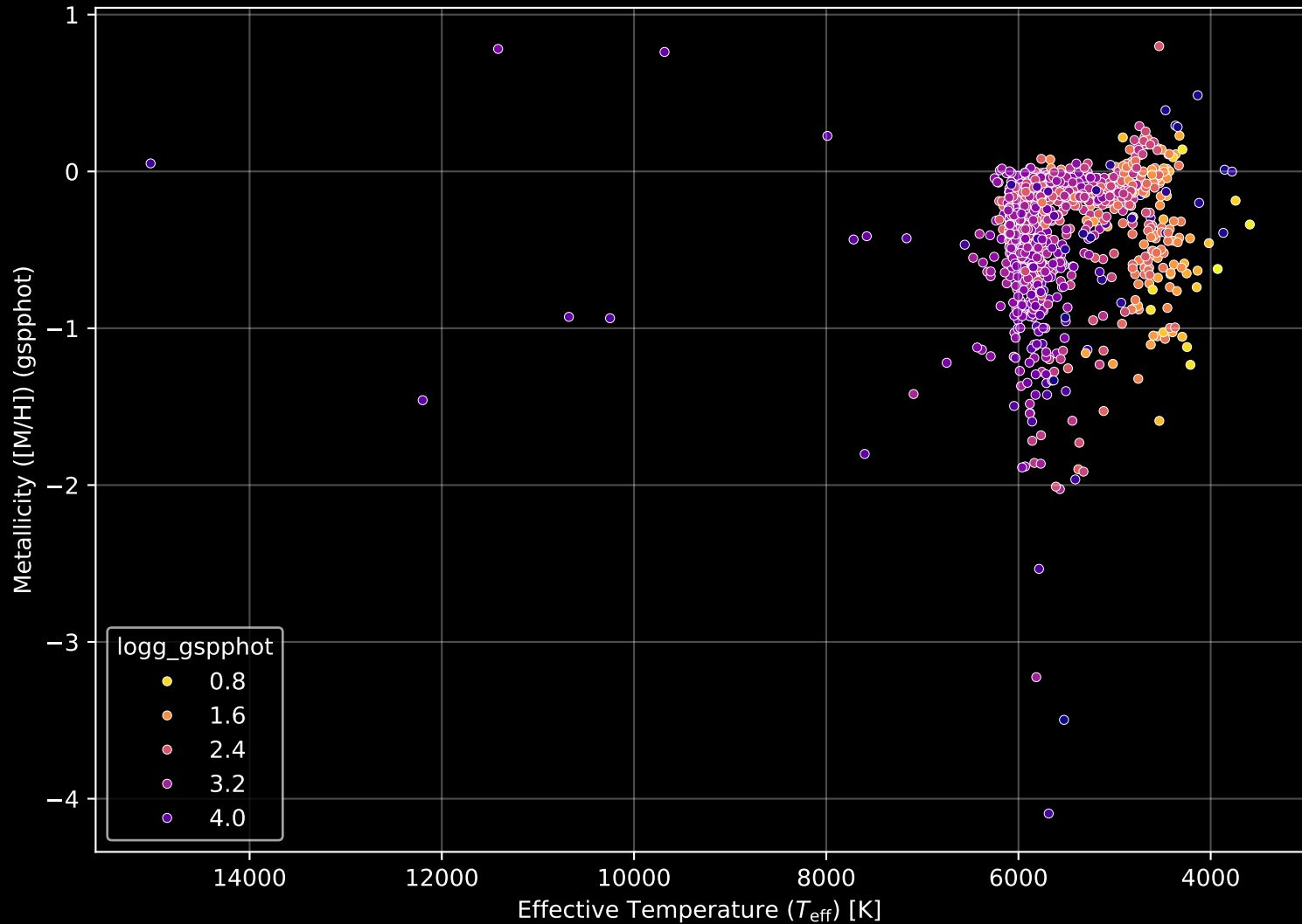
APOGEE DR17 Field: [Omgacen] Stellar Population Parameters (n= 1069)
